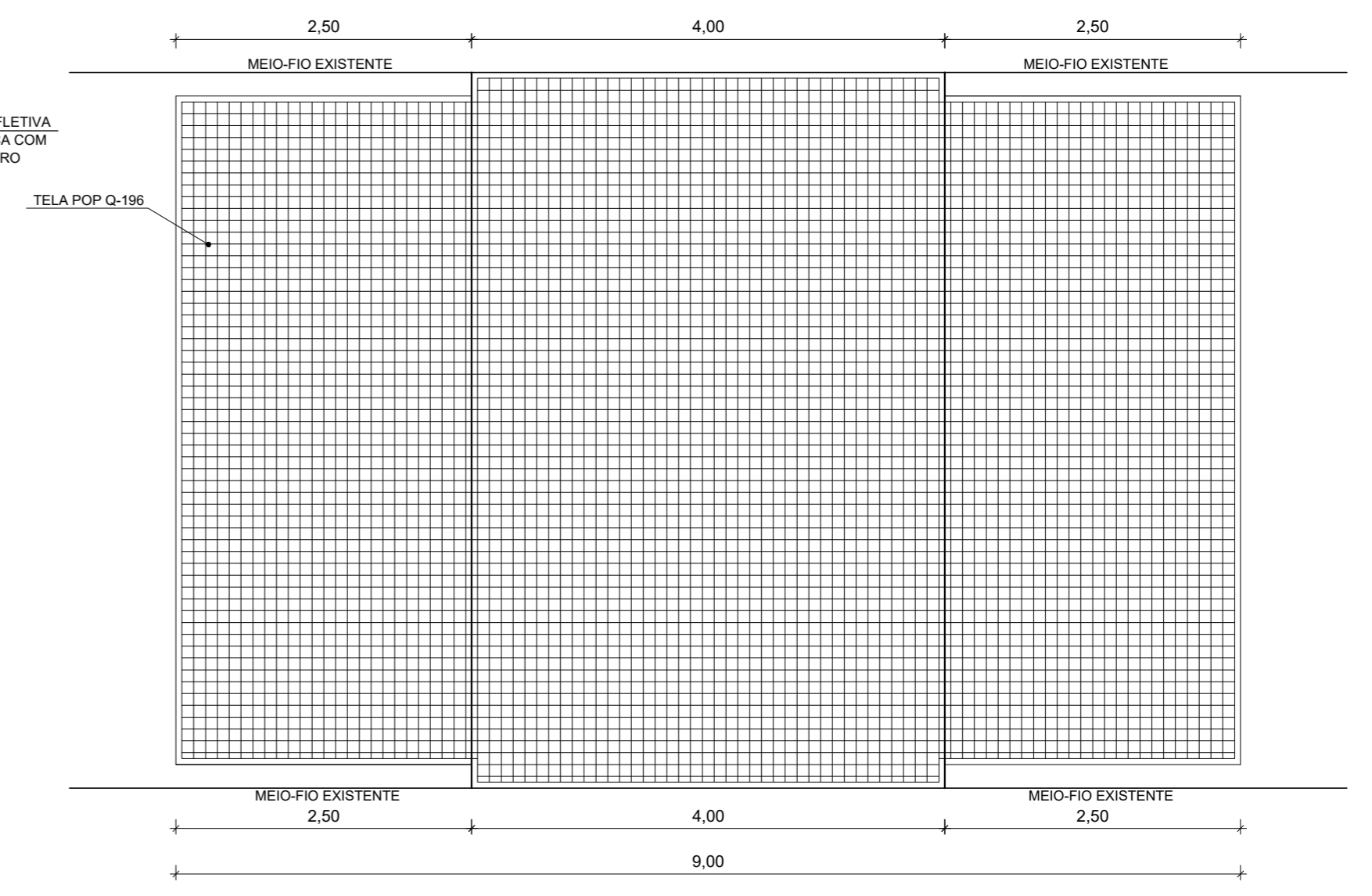
18 ARMADURA DE RADIER ESC.: 1/50
