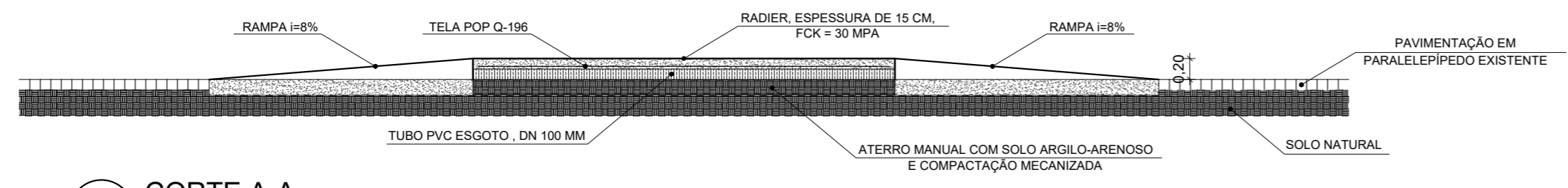
16 CORTE A-A ESC.: 1/50
