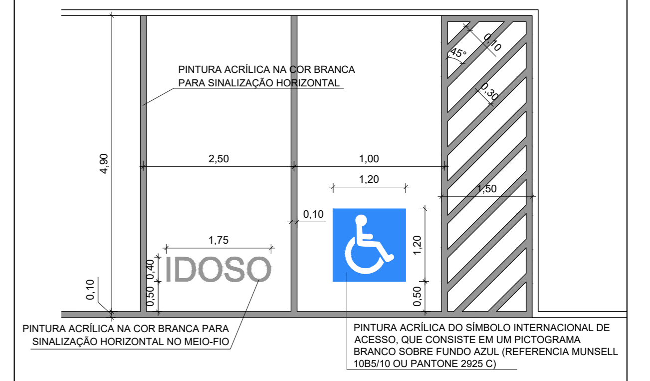
19 DETALHE DA SINALIZAÇÃO HORIZONTAL SEM ESCALA
