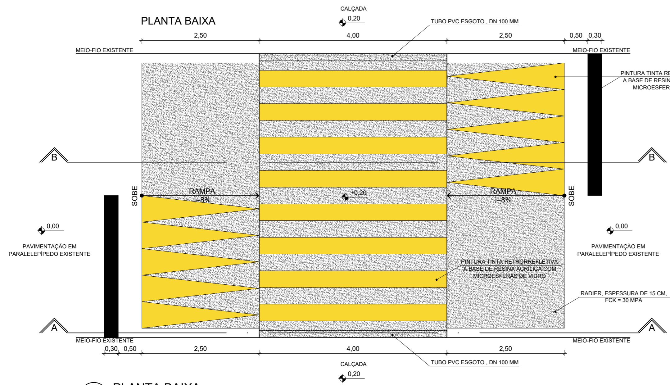
15 PLANTA BAIXA ESC.: 1/50
