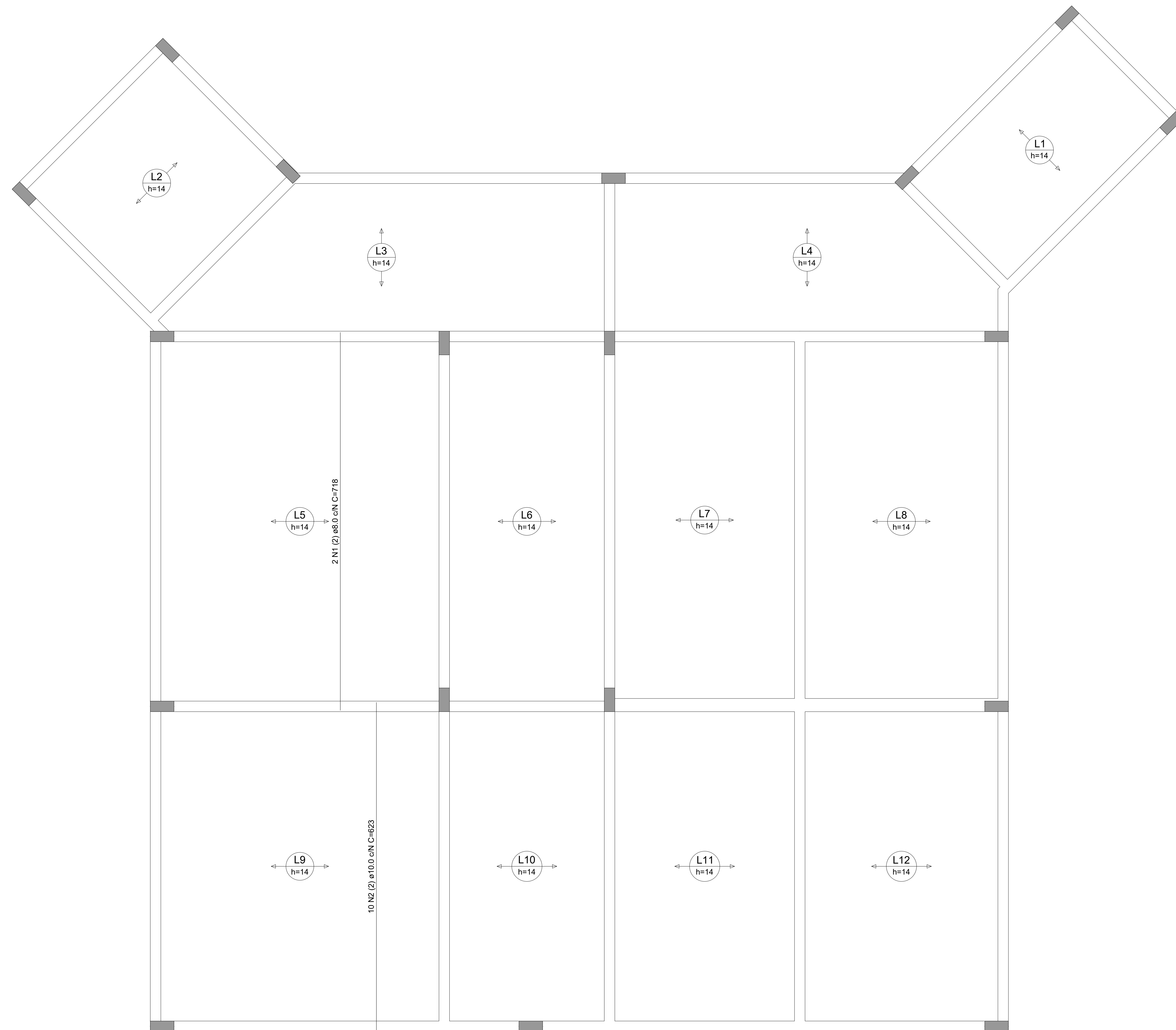
Armação positiva das lajes do pavimento Coberta (Eixo Y) escala 1:50
