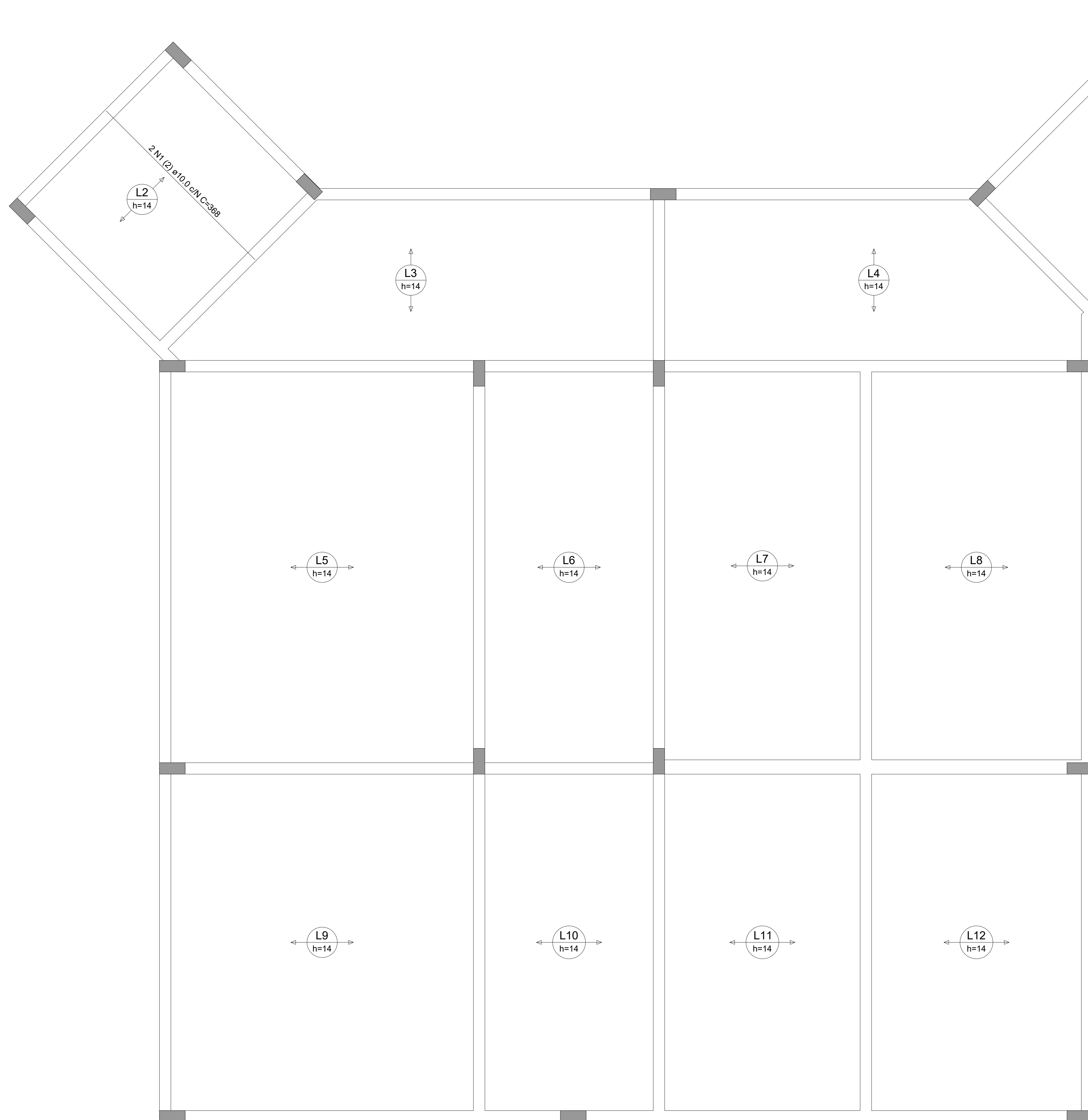
Armação positiva das lajes do pavimento Coberta (Eixo X) escala 1:50
